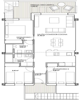
planta primera Sup. Construida VV.V. = 80,46 m²
