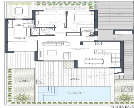
PLANTA BAJA
