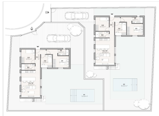
PLANTA BAJA S. COMERCIAL 10.00m 2 S. VIV. 80.00m 2 S. VIV. 10.00m 2 S. VIV. 10.00m 2
