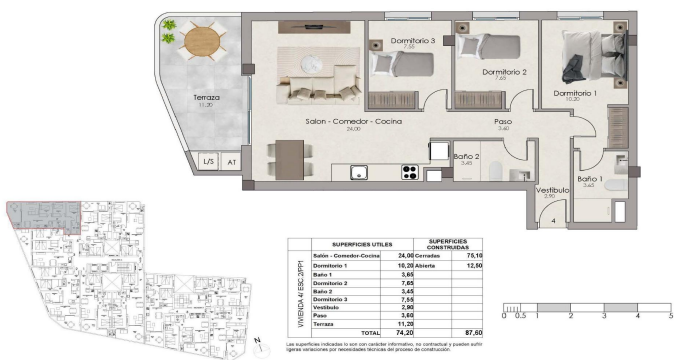
PLANTA PISO 1 / ESCALERA 2 VIVIENDA 4
