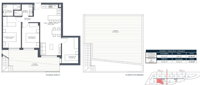
E: 1/100. Vivienda Esc.1-Ático-B
