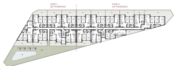
E: 1/350. Planta Primera
